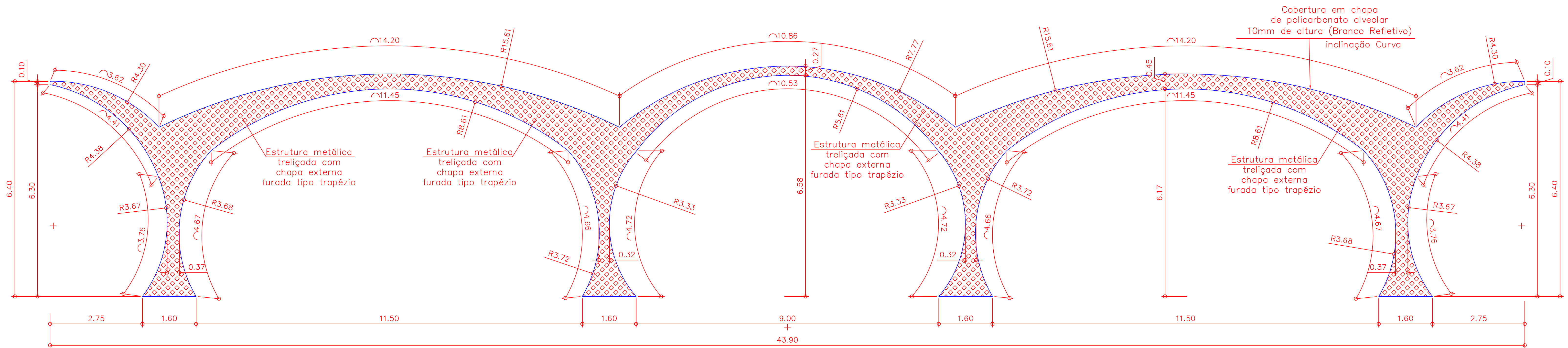
4 DETALHAMENTO PÓRTICO Esc. 1:50
